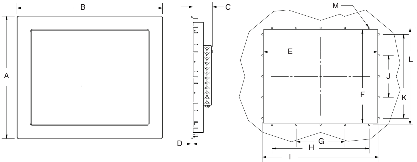
Cutout Dimensions
